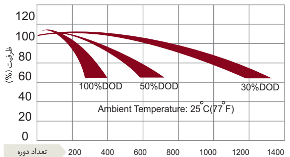
طول چرخه عمر نسبت به عمق دشارژ
